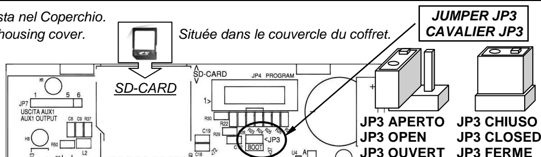
Fig.8-Inserimento SD-Card
