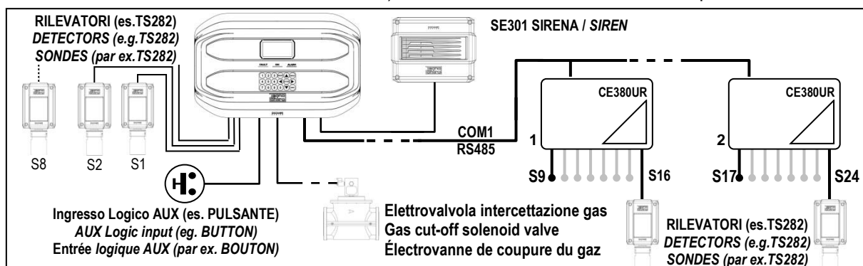
Fig.2 - Par ex. schéma d'installation avec des détecteurs de la série TS282.
