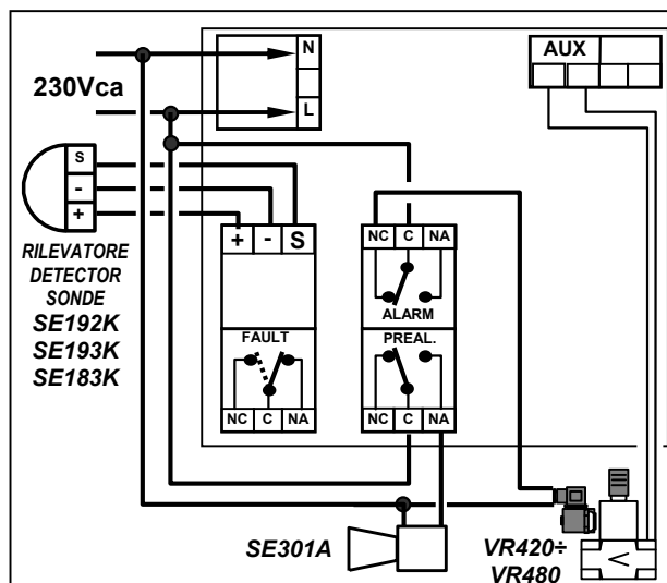
Fig. 5 Collegamento con valvola a riarmo manuale Norm.Chiusa Wiring diagram with a normally closed manual resetting valve Schéma avec vanne à réarmement manuel norm. fermée Esquema con válvula de rearmado manual norm. cerrada
