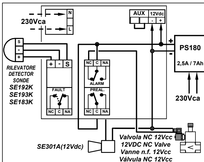
Fig. 6 Collegamento 12Vcc con valvola a riarmo man. Norm.Chiusa 12Vdc Wiring diagram with a normally closed manual resetting valve Schéma à 12Vcc avec vanne à réarmement manuel norm. Fermée Esquema de 12Vdc con válvula de rearmado manual norm. cerrada
